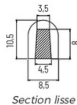
Section lisse
